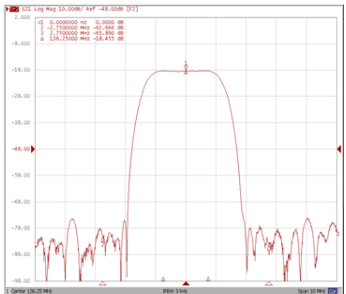
Attenuation Fo±2.75MHz
