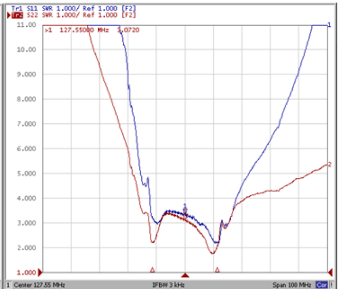
VSWR
