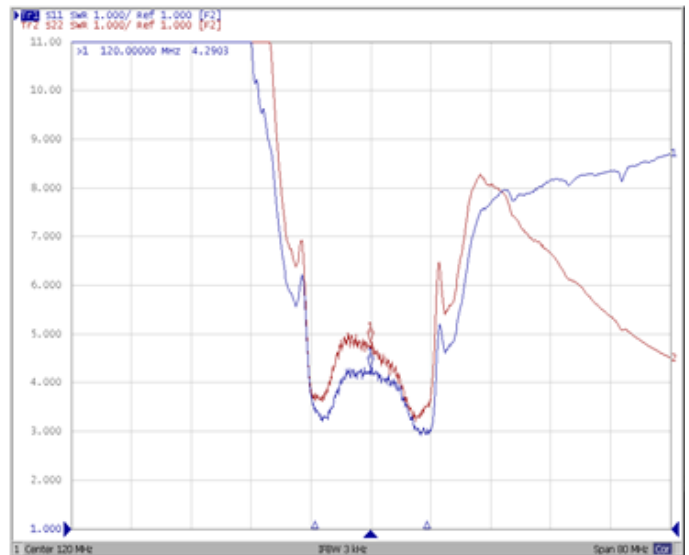
VSWR
