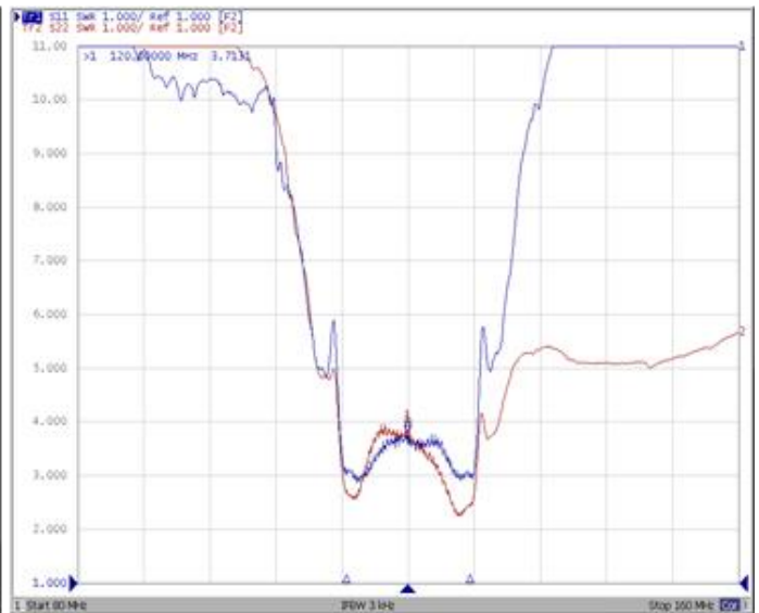
VSWR
