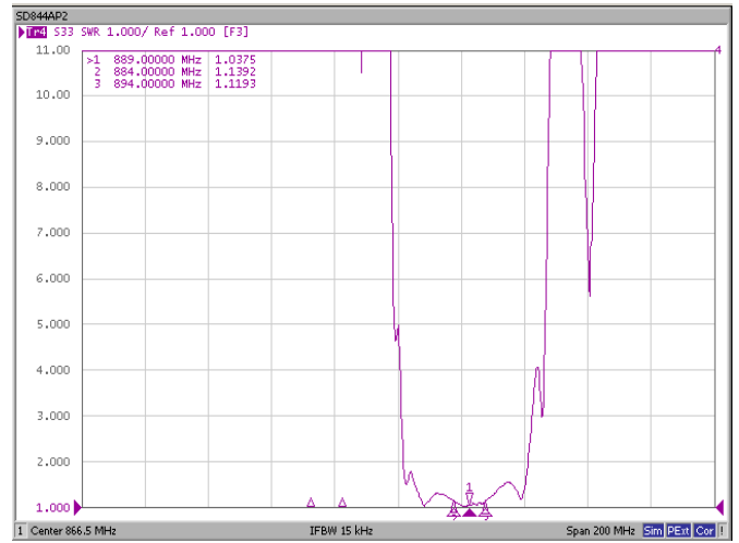
VSWR
