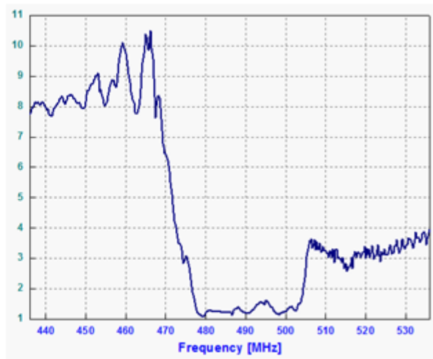
VSWR
