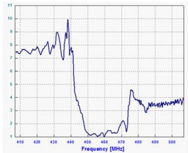
VSWR
